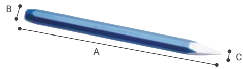
► PUNTERO OCTOGONAL 5821
